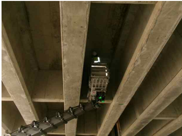
고소작업차를 이용한 근접조사
